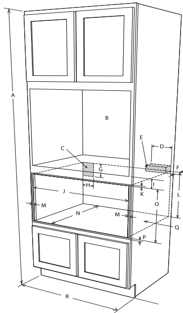
Dimensions de la découpe 28 7/16 po x 15 9/16 po (722,31 x 395,27 mm)
