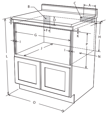
Dimensions de la découpe 28 7/16 po x 15 9/16 po (722,31 x 395,27 mm)
